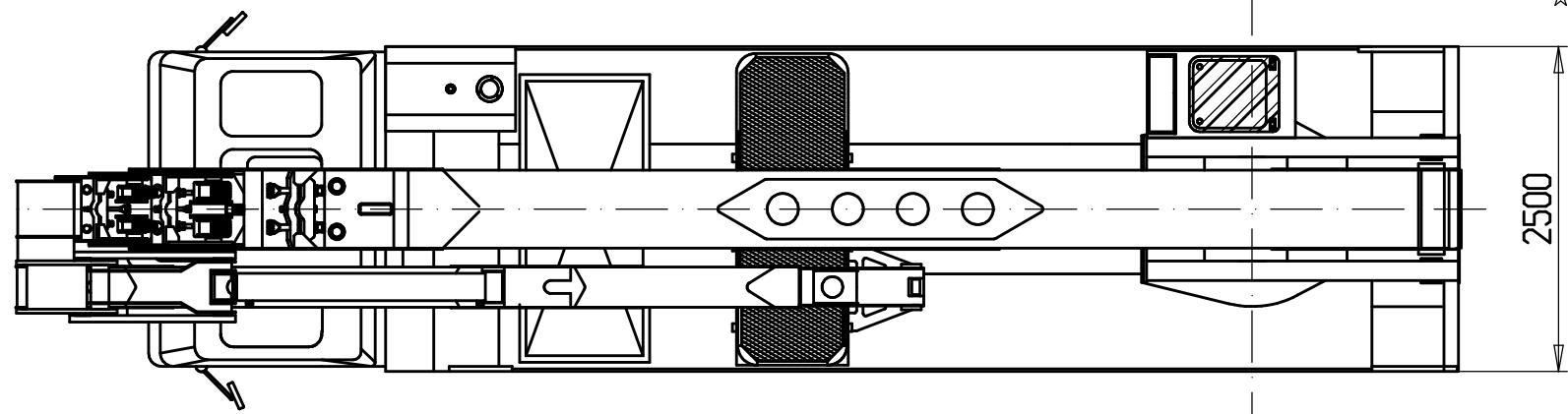
DISEGNO: Installazione "EAGLE 5227/30" su SCANIA P124 CB 8X4 HZ 420
